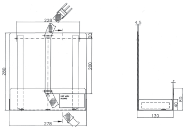
PNR 6240-37 • Bracket
