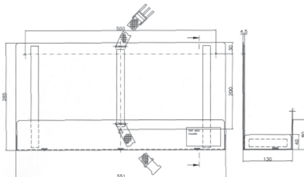
PNR 6240-01-001 • Bracket
