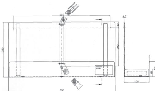
PNR 6240-01-001 • Bracket
