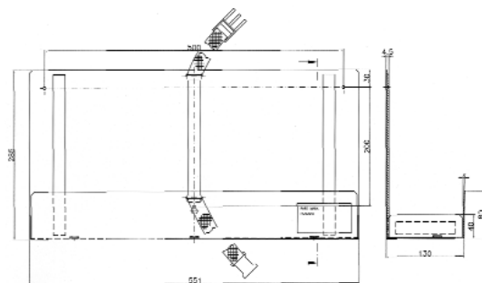
PNR 6240-01-001 • Bracket
