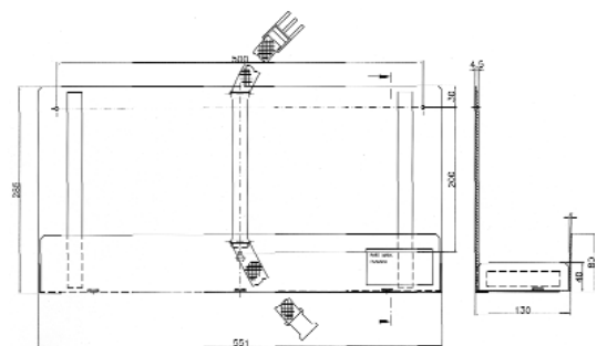
PNR 6240-01-001 • Bracket
