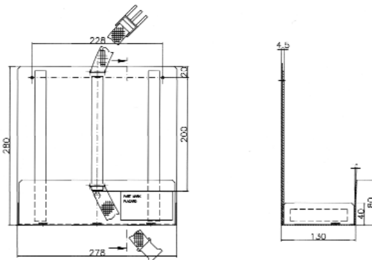
PNR 6240-37-011 • Bracket
